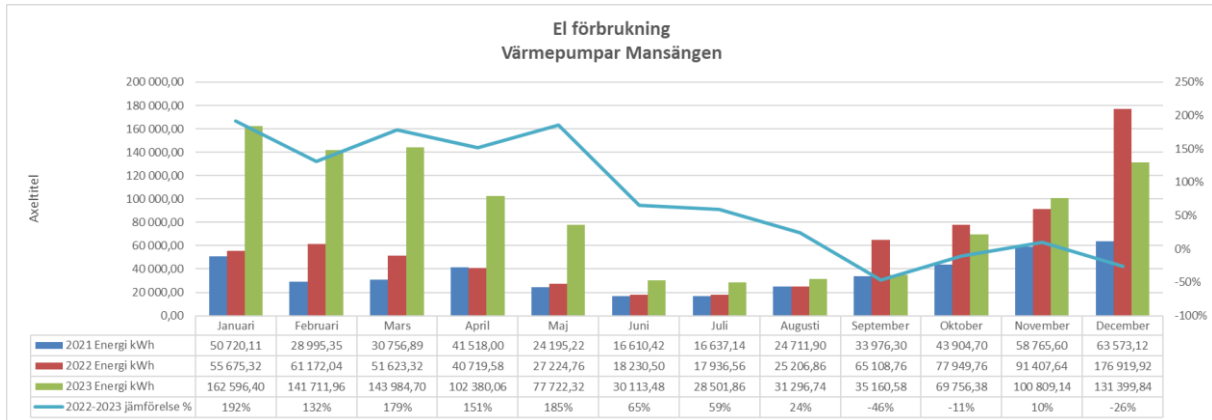
Figur 5 – Elförbrukning värmepumpar Mansängen 2023
