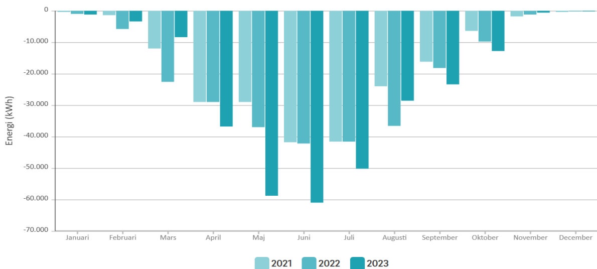
Figur 6 – Producerad solel som gått ut på elnätet 2021-2023
