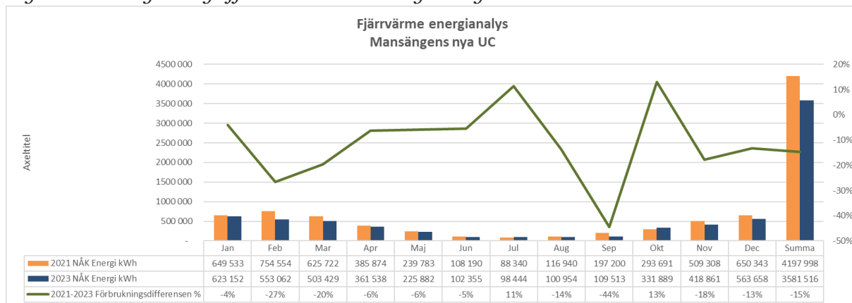
Figur 2 – Energianalys fjärrvärme Mansängens nya undercentral
